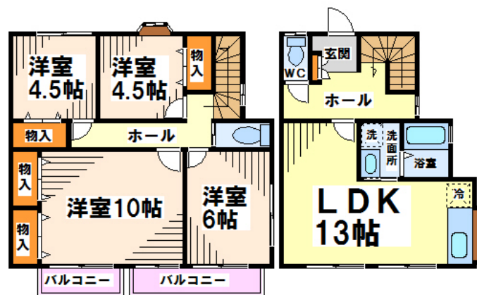
【間取り図】
